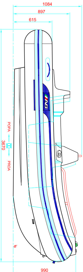
LONGITUDINAL PROFILE
