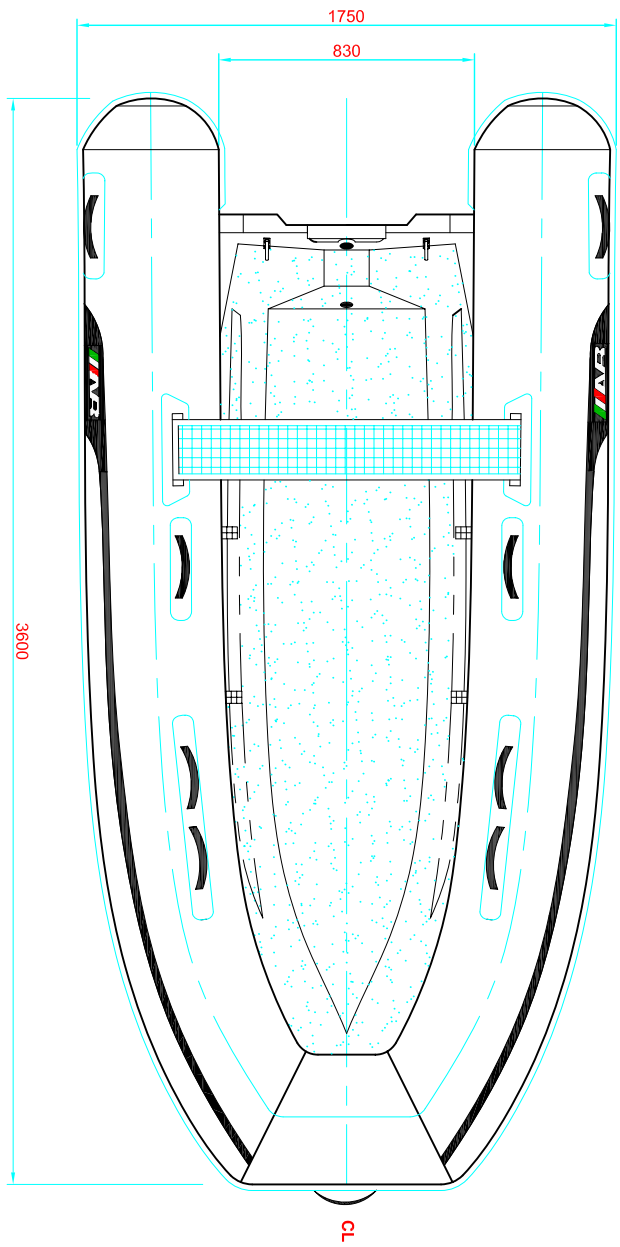
PLANT VIEW VISTA EN PLANTA
