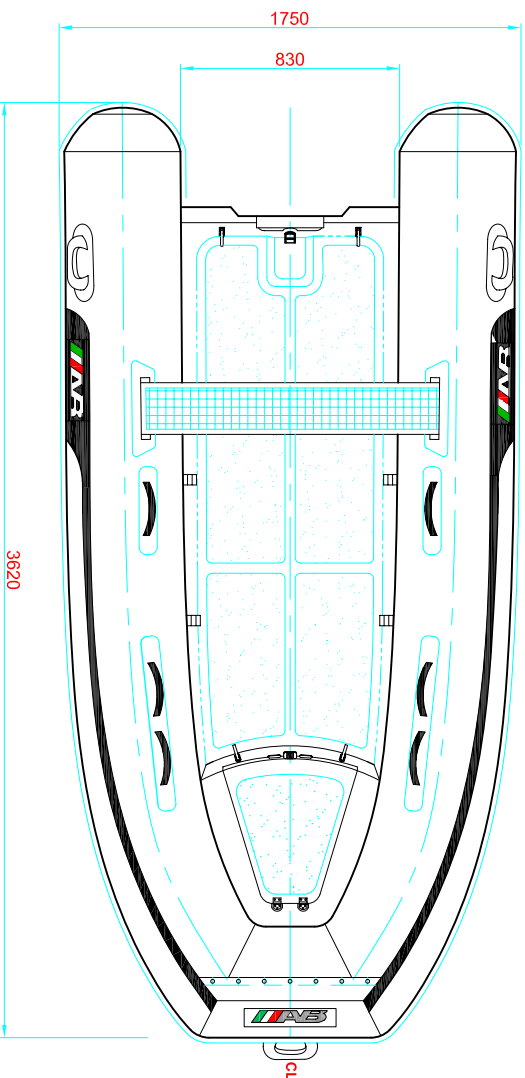
PLANT VIEW VISTA EN PLANTA
