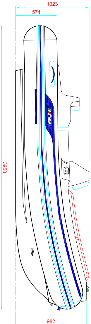
LONGITUDINAL PROFILE
