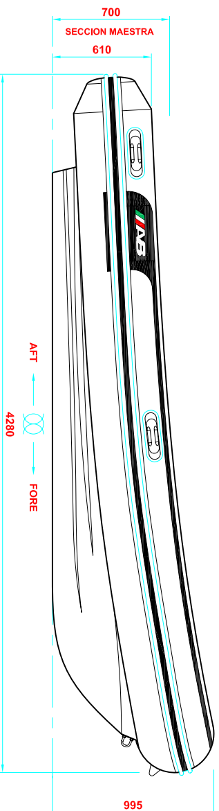
LONGITUDINAL PROFILE PERFIL LONGITUDINAL
