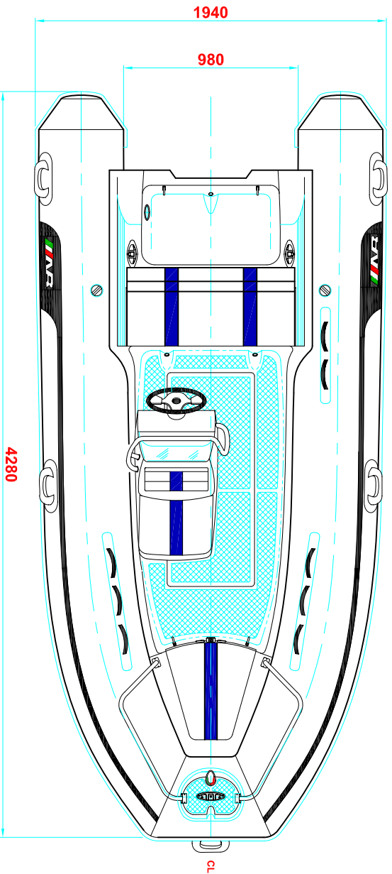
PLANT VIEW VISTA EN PLANTA
