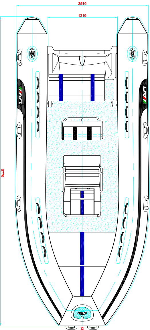
PLANT VIEW VISTA EN PLANTA
