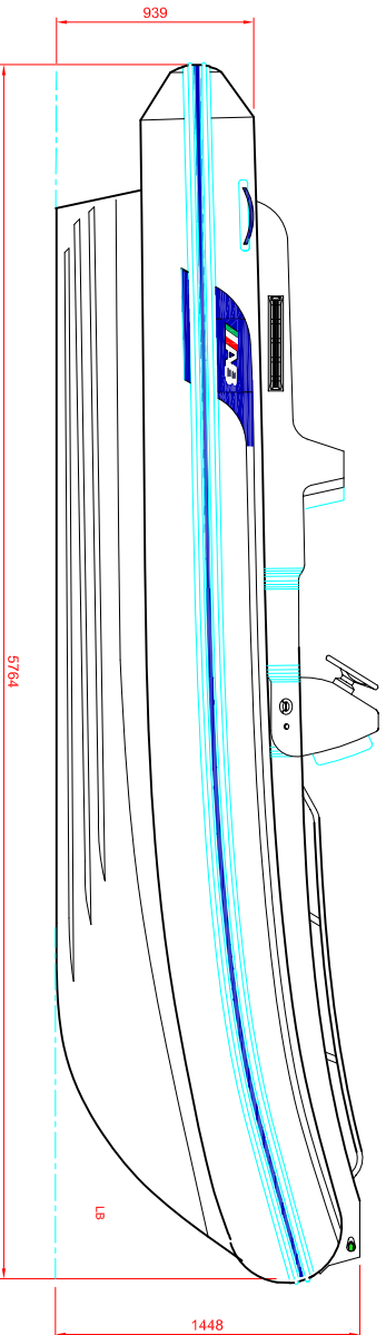
LONGITUDINAL PROFILE
