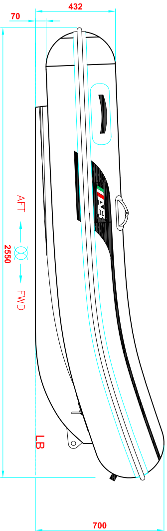
LONGITUDINAL PROFILE PERFIL LONGITUDINAL
