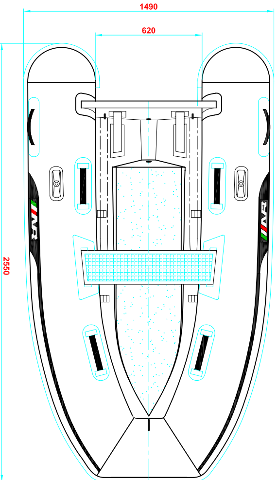
PLANT VIEW VISTA EN PLANTA
