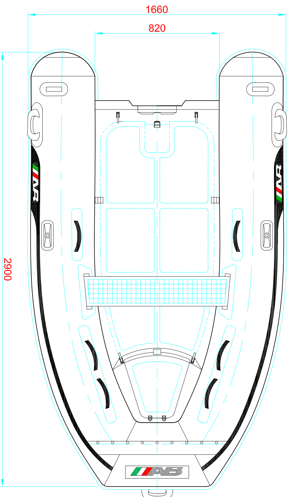
PLANT VIEW VISTA EN PLANTA
