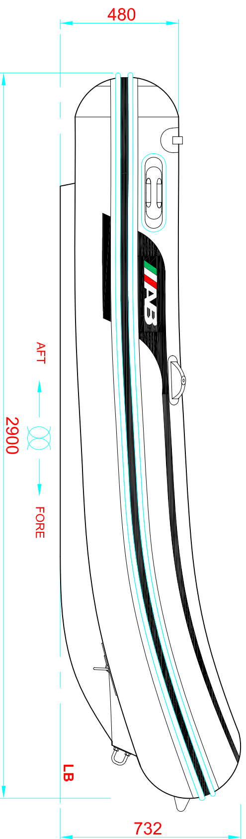
LONGITUDINAL PROFILE PERFIL LONGITUDINAL
