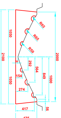
TRANSVERSAL SECTION "B" SECCION TRANSVERSAL "B"
