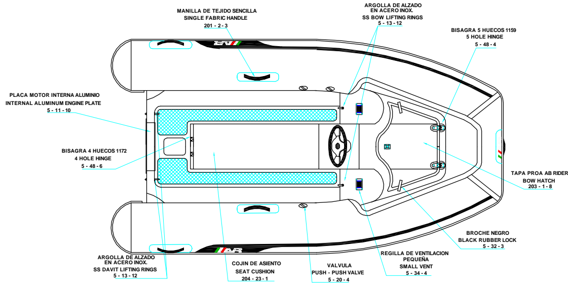
PLANT VIEW VISTA EN PLANTA
