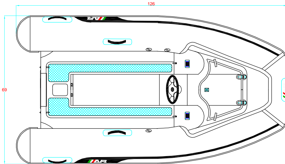
PLANT VIEW VISTA EN PLANTA
