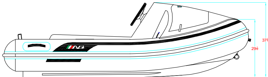
LONGITUDINAL PROFILE VISTA LATERAL
