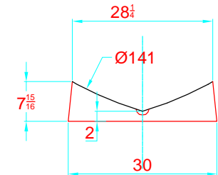
TRANSVERSAL SECTION "B" SECCION TRANSVERSAL "B"
