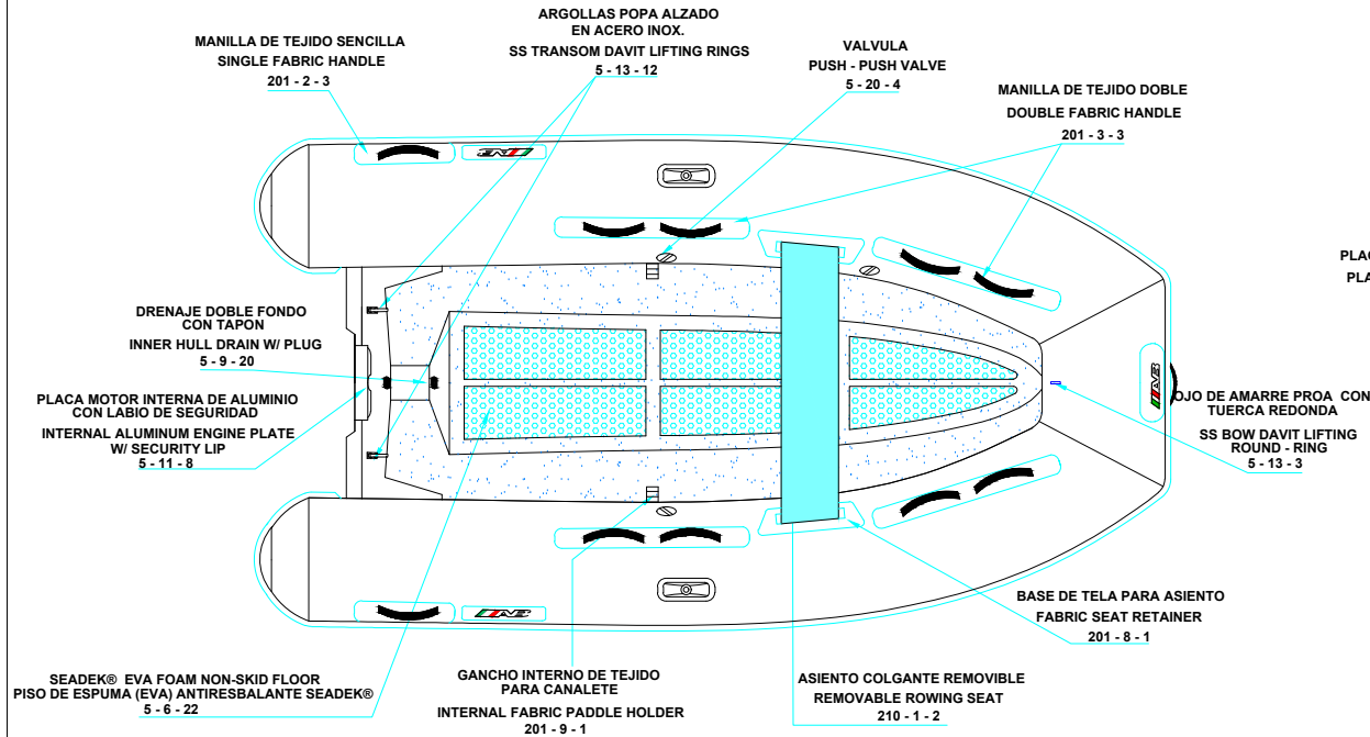
PLANT VIEW VISTA EN PLANTA
