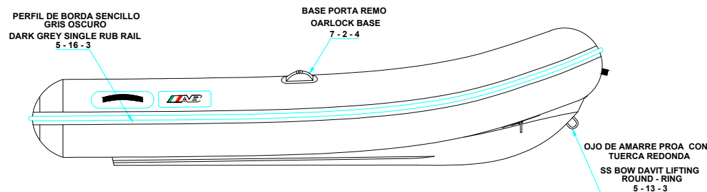
LONGITUDINAL PROFILE VISTA LATERAL
