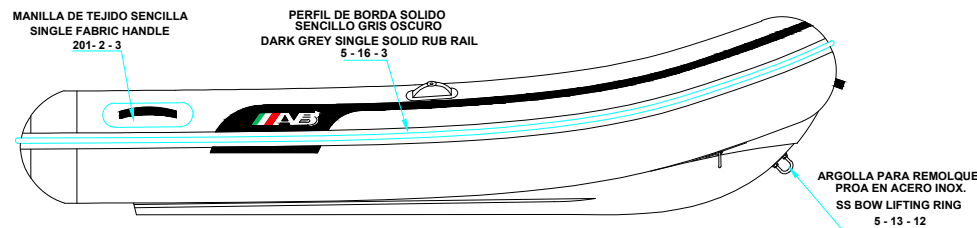
LONGITUDINAL PROFILE VISTA LATERAL
