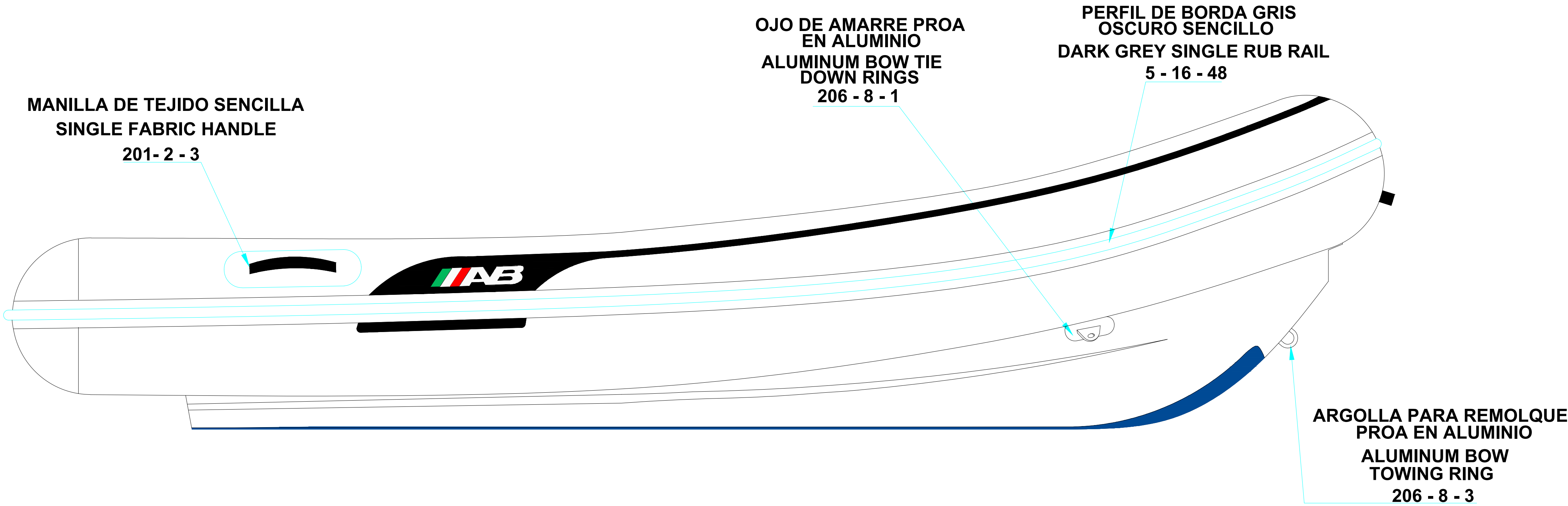
LONGITUDINAL PROFILE VISTA LATERAL
