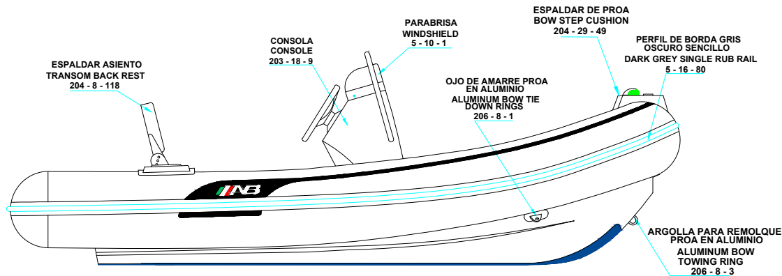
LONGITUDINAL PROFILE VISTA LATERAL
