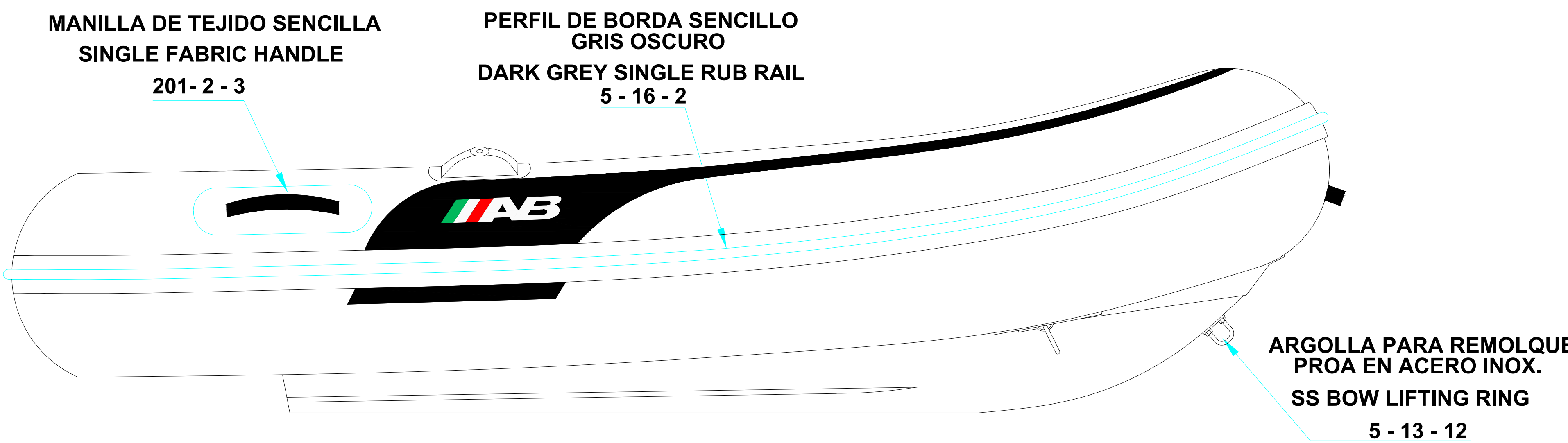
LONGITUDINAL PROFILE VISTA LATERAL
