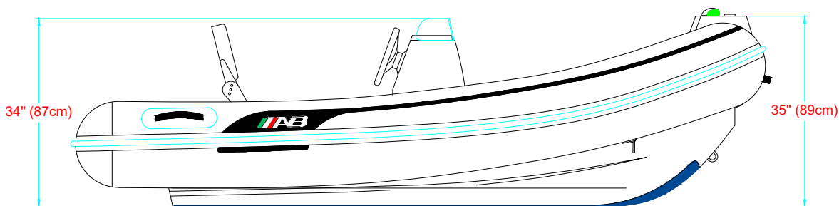
LONGITUDINAL PROFILE VISTA LATERAL
