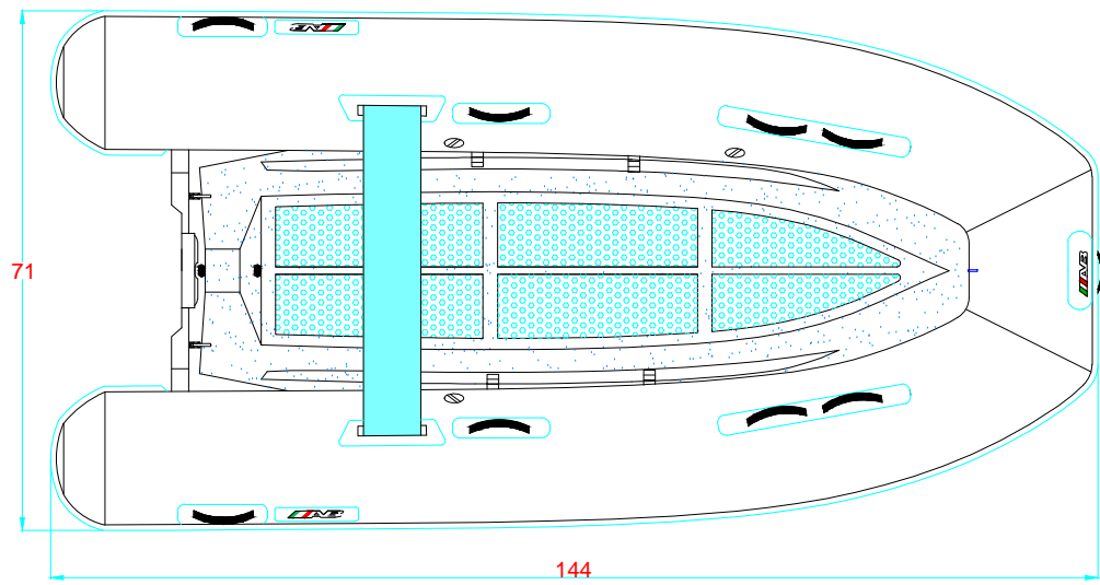
PLANT VIEW VISTA EN PLANTA
