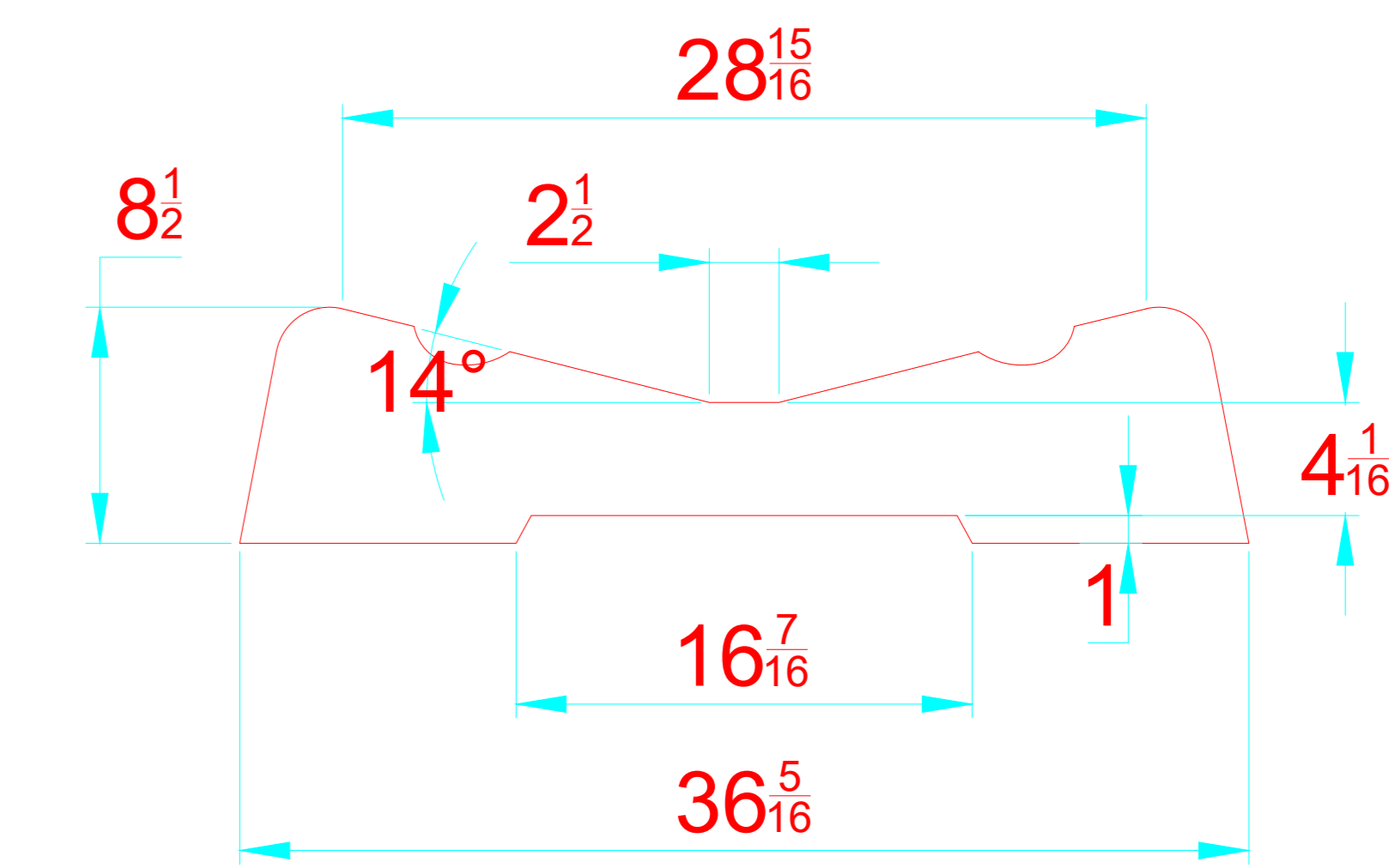
TRANSVERSAL SECTION "B" SECCION TRANSVERSAL "B"
