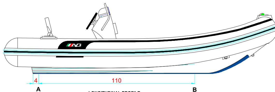
LONGITUDINAL PROFILE PERFIL LONGITUDINAL
