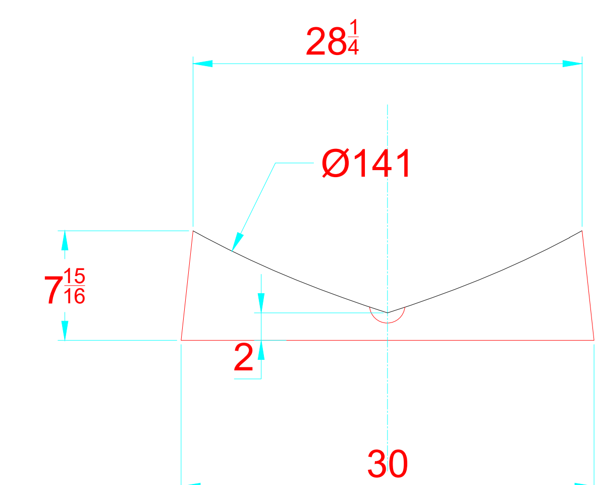
TRANSVERSAL SECTION "B" SECCION TRANSVERSAL "B"
