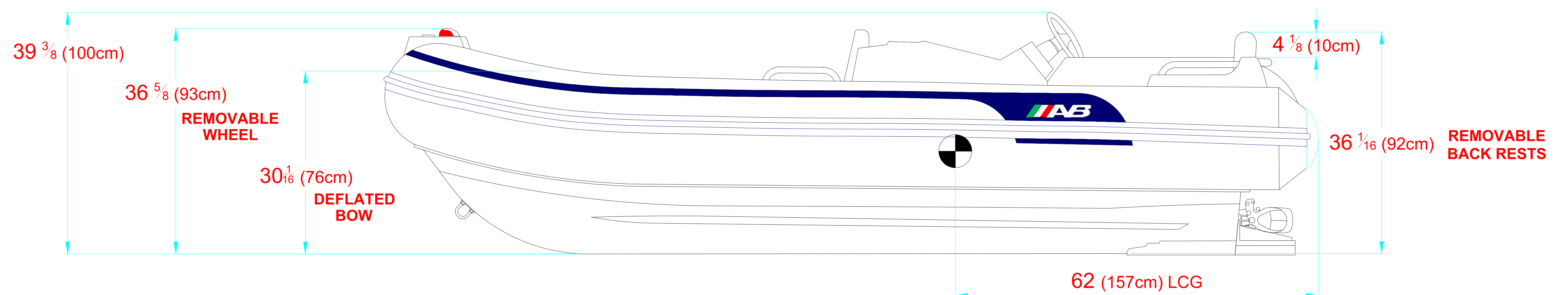
LONGITUDINAL PROFILE VISTA LATERAL
