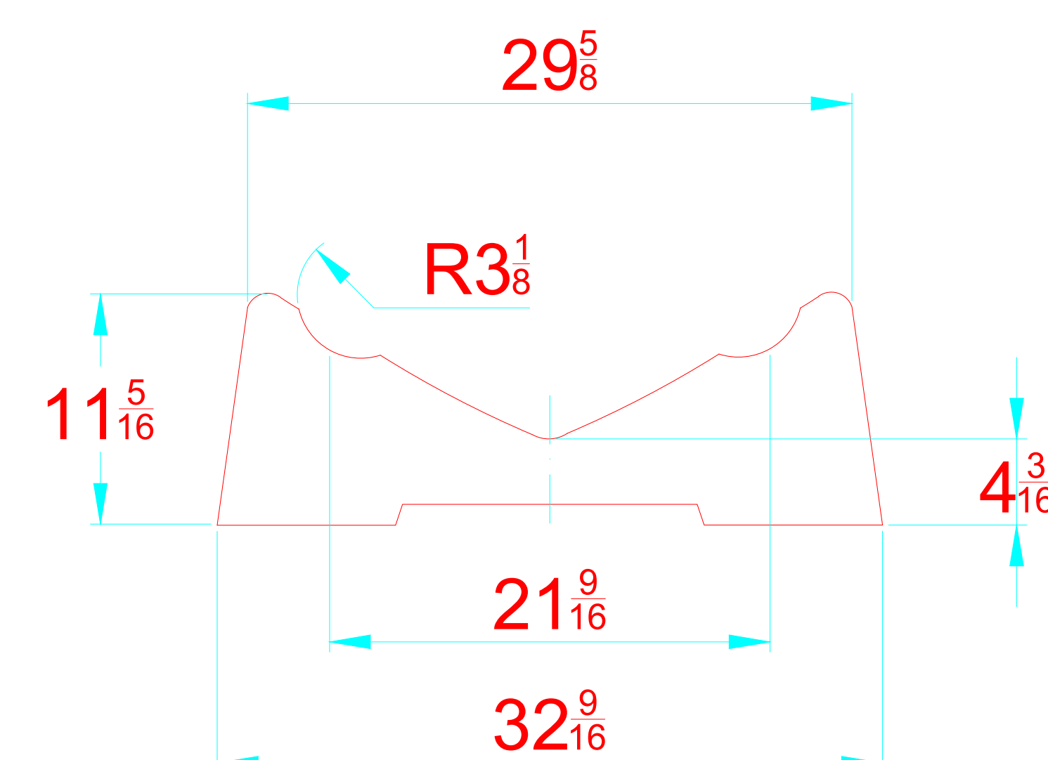
TRANSVERSAL SECTION "B" SECCION TRANSVERSAL "B"
