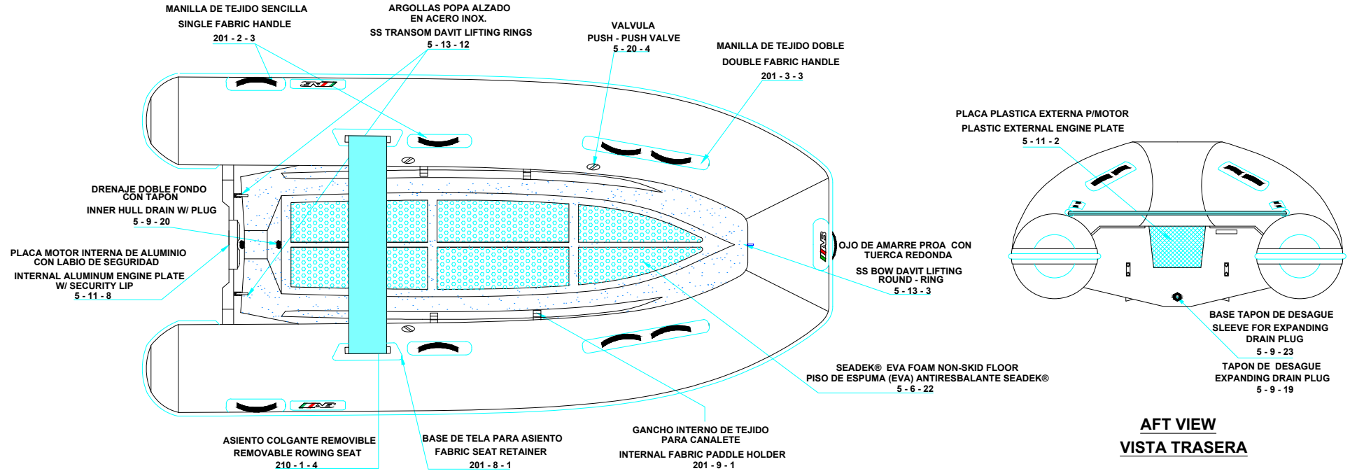
PLANT VIEW VISTA EN PLANTA
