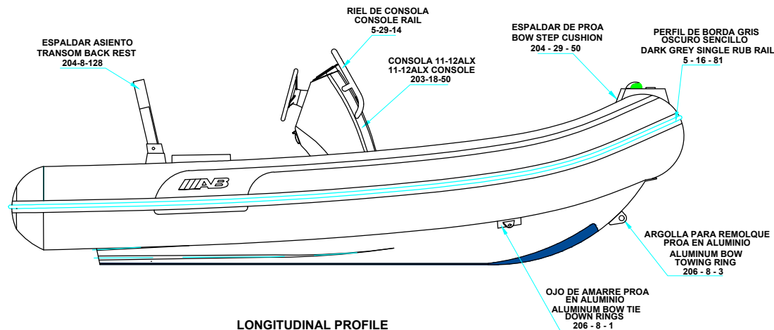
LONGITUDINAL PROFILE VISTA LATERAL
