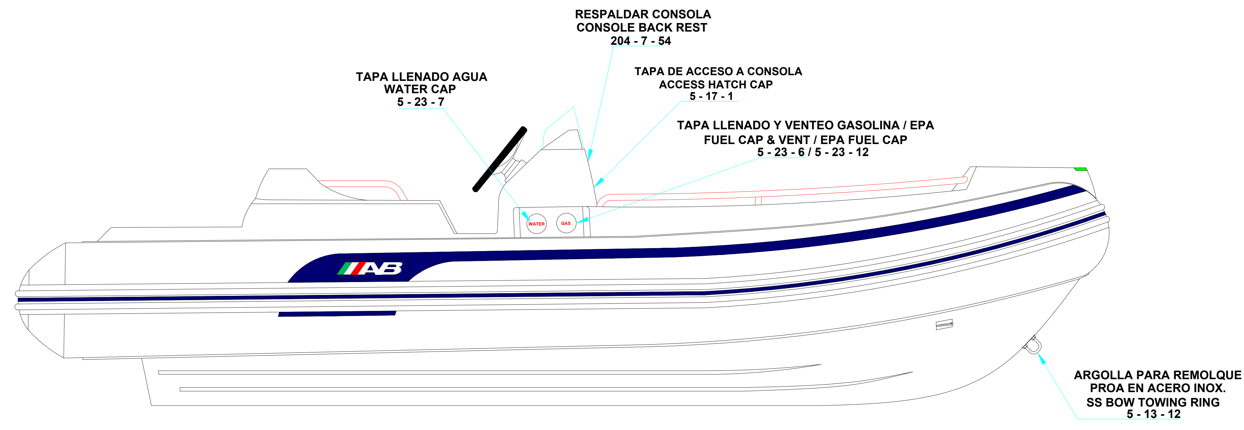
LONGITUDINAL PROFILE VISTA LATERAL
