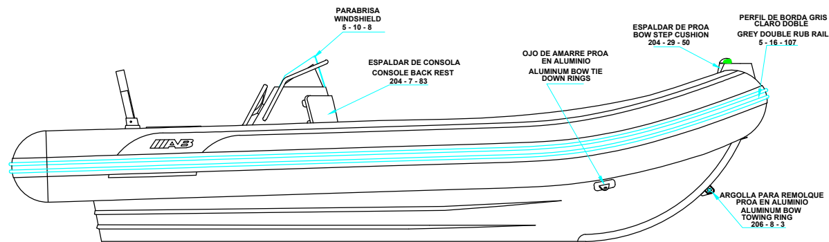
LONGITUDINAL PROFILE VISTA LATERAL
