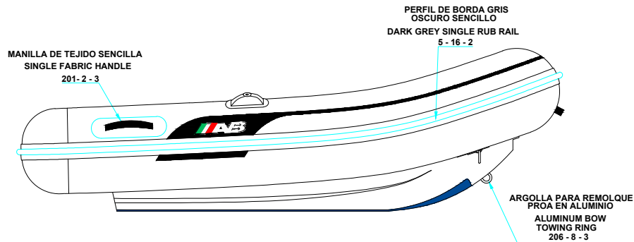
LONGITUDINAL PROFILE VISTA LATERAL
