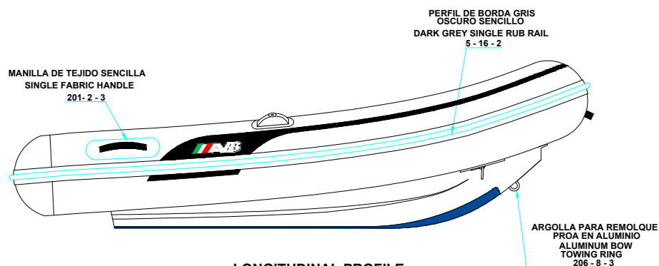
LONGITUDINAL PROFILE VISTA LATERAL
