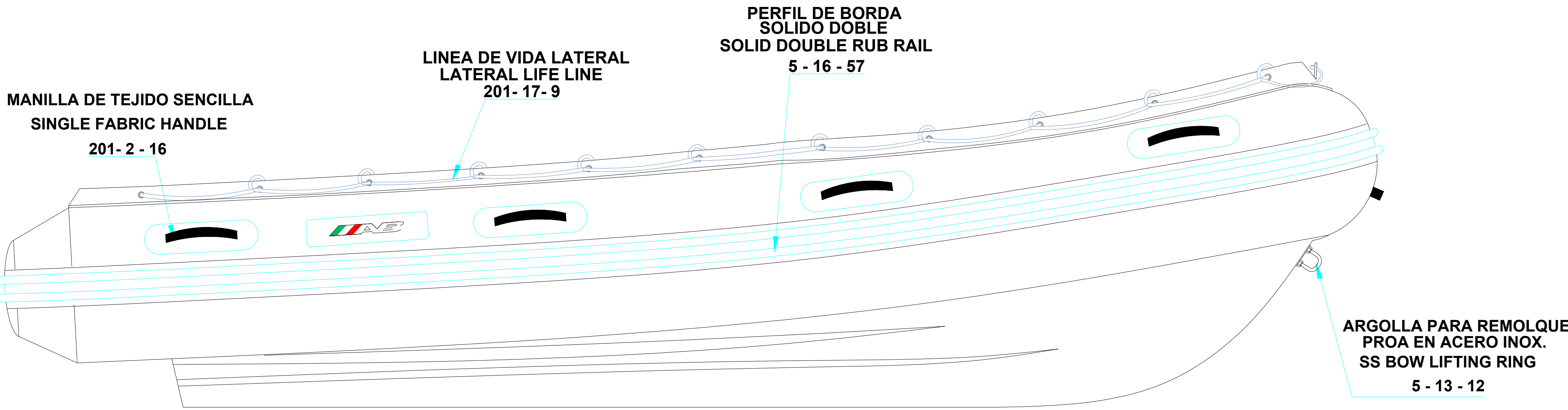
LONGITUDINAL PROFILE VISTA LATERAL
