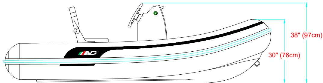
LONGITUDINAL PROFILE VISTA LATERAL
