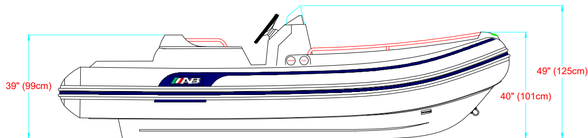
LONGITUDINAL PROFILE VISTA LATERAL
