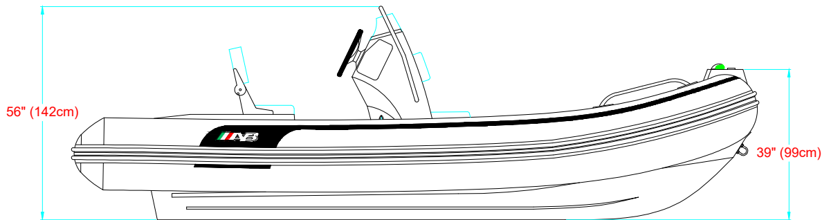
LONGITUDINAL PROFILE VISTA LATERAL
