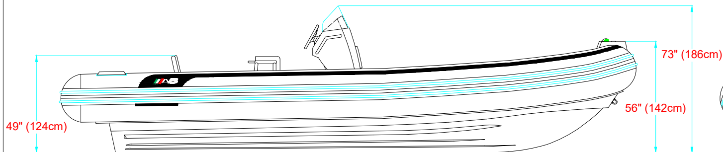
LONGITUDINAL PROFILE VISTA LATERAL
