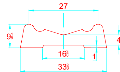
TRANSVERSAL SECTION "B" SECCION TRANSVERSAL "B"
