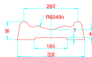
TRANSVERSAL SECTION "B" SECCION TRANSVERSAL "B"
