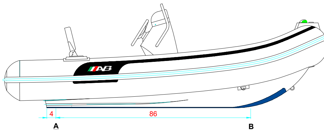
LONGITUDINAL PROFILE PERFIL LONGITUDINAL
