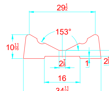
TRANSVERSAL SECTION "B" SECCION TRANSVERSAL "B"
