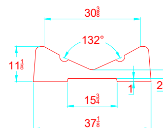
TRANSVERSAL SECTION "B" SECCION TRANSVERSAL "B"
