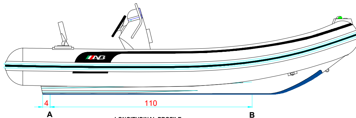
LONGITUDINAL PROFILE PERFIL LONGITUDINAL
