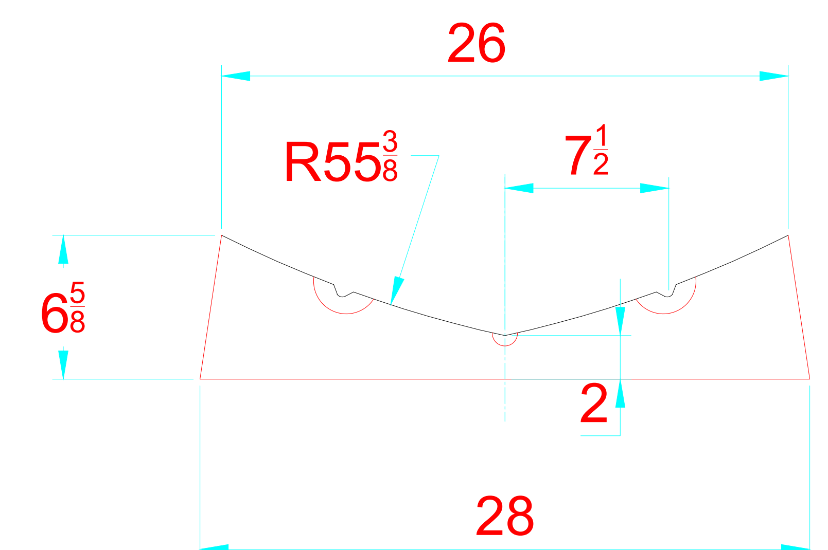
TRANSVERSAL SECTION "B" SECCION TRANSVERSAL "B"
