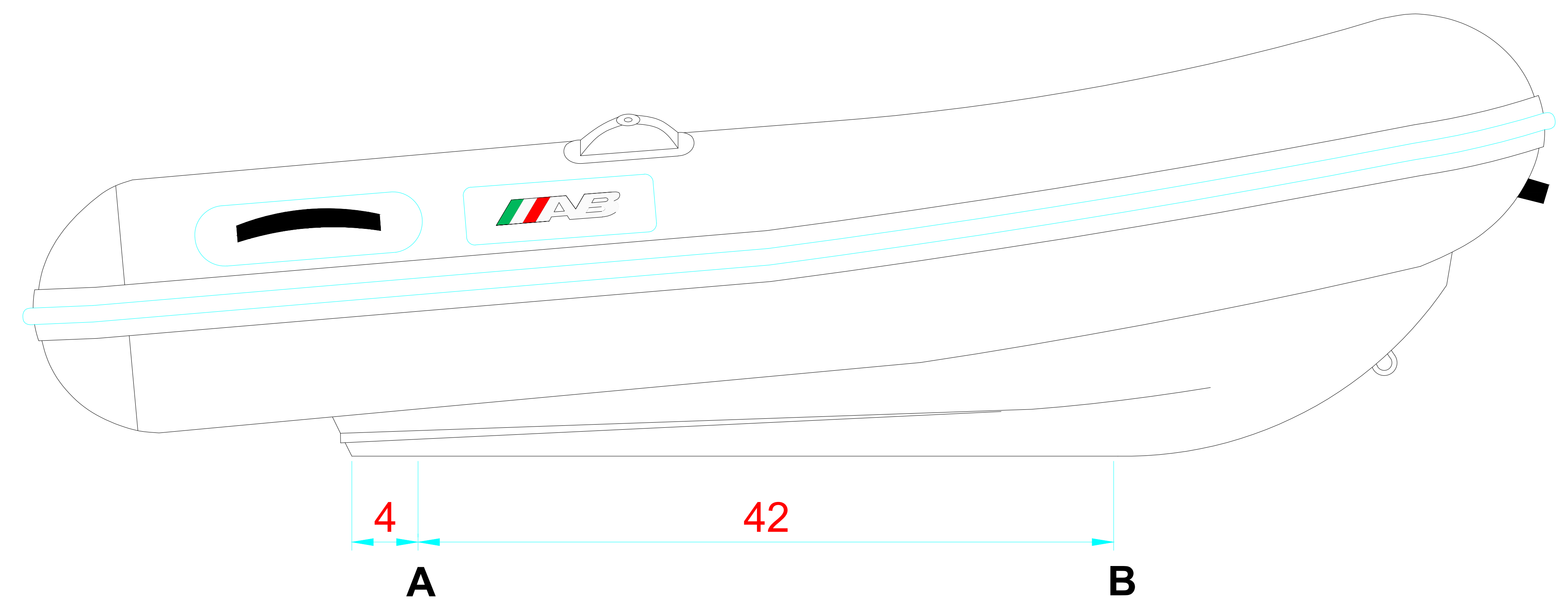
LONGITUDINAL PROFILE PERFIL LONGITUDINAL
