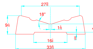
TRANSVERSAL SECTION "B" SECCION TRANSVERSAL "B"
