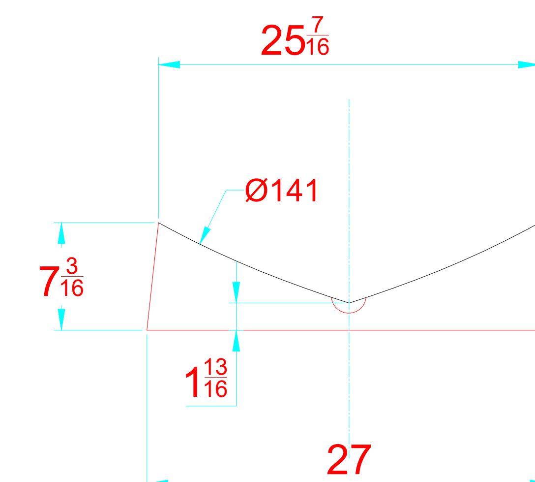
TRANSVERSAL SECTION "B" SECCION TRANSVERSAL "B"
