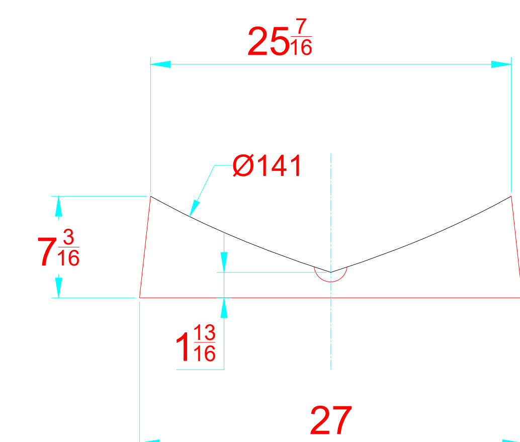
TRANSVERSAL SECTION "B" SECCION TRANSVERSAL "B"
