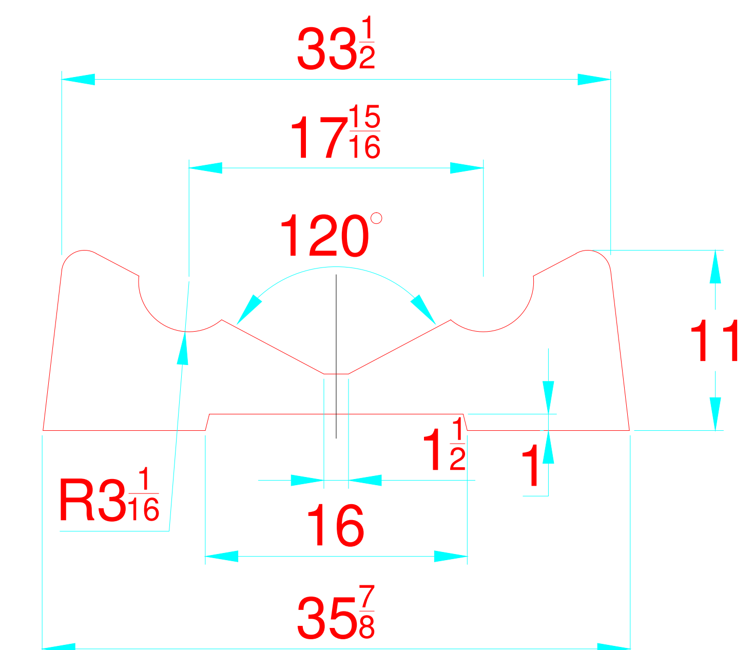
TRANSVERSAL SECTION "B" SECCION TRANSVERSAL "B"
