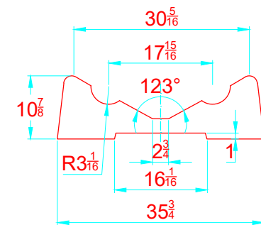
TRANSVERSAL SECTION "B" SECCION TRANSVERSAL "B"
