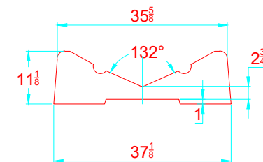
TRANSVERSAL SECTION "B" SECCION TRANSVERSAL "B"
