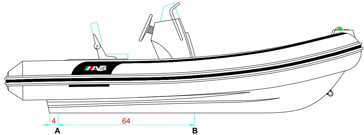
LONGITUDINAL PROFILE VISTA LATERAL
